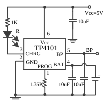
TP4101 单灯 0.6A 充电电池管理电路
