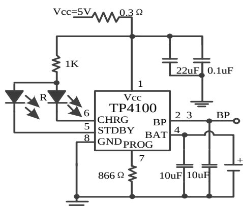
TP4100 带耗散电阻 双灯 1A 充电电池管理电路
