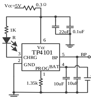
TP4101 带耗散电阻 单灯 0.6A 充电电池管理电路
