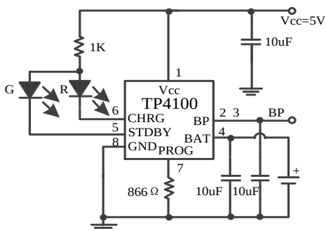
TP4100 双灯 1A 充电电池管理电路
